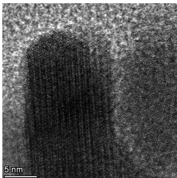
Fig S1: TEM images of LSF@20B 2 O 3 .
