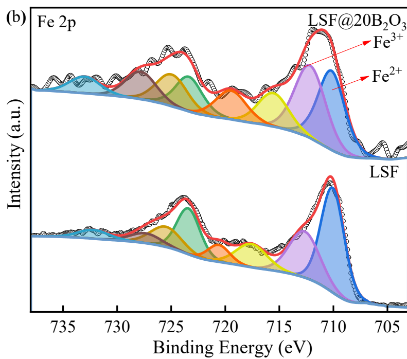
Fig S2: Fe 2p XPS spectra.
